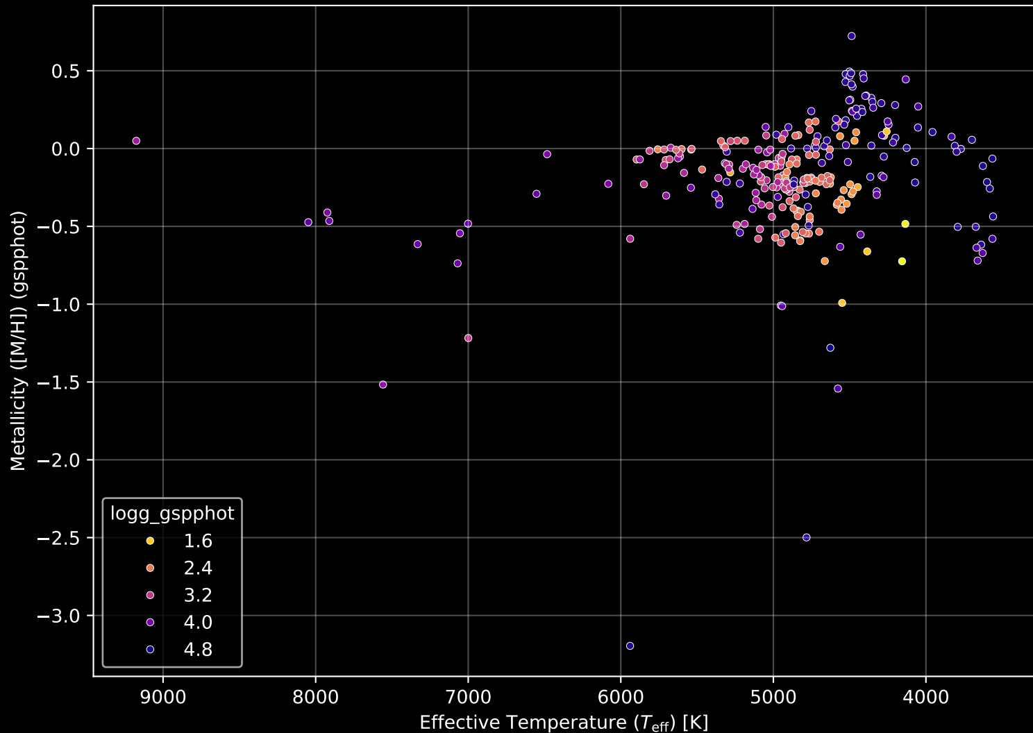
APOGEE DR17 Field: [232+30_btx] Stellar Population Parameters (n= 283)
